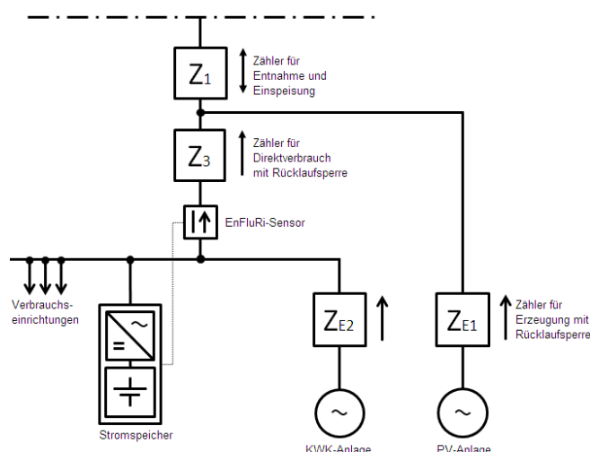
Speicherschema 22
