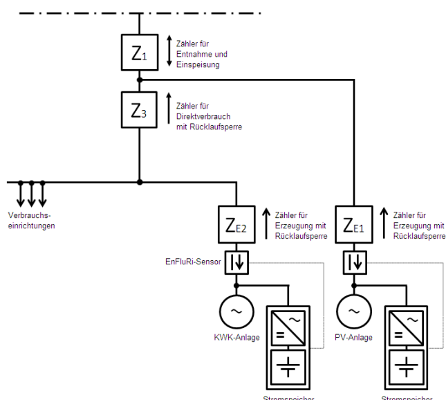
Speicherschema 12
