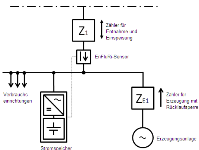
Speicherschema 13
